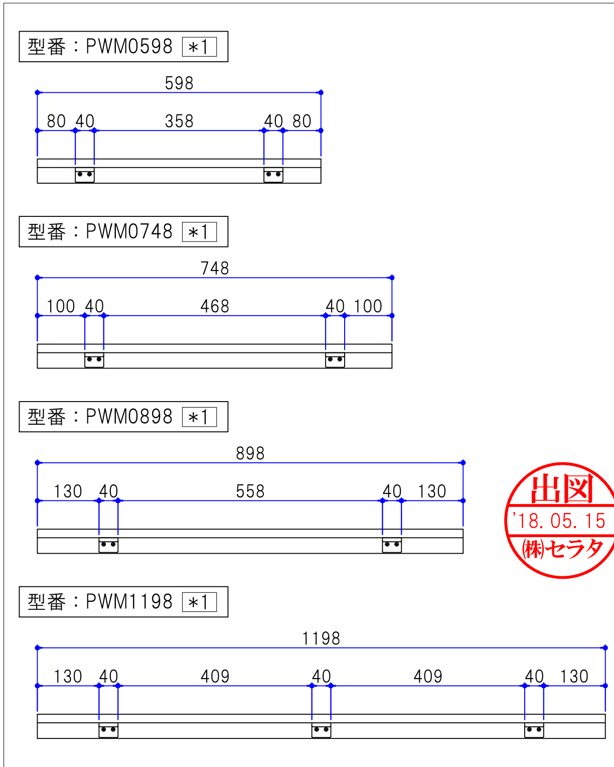
② 金具取付位置参照図 (1/8)
