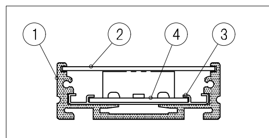
A-A 断面図 (1/1)
